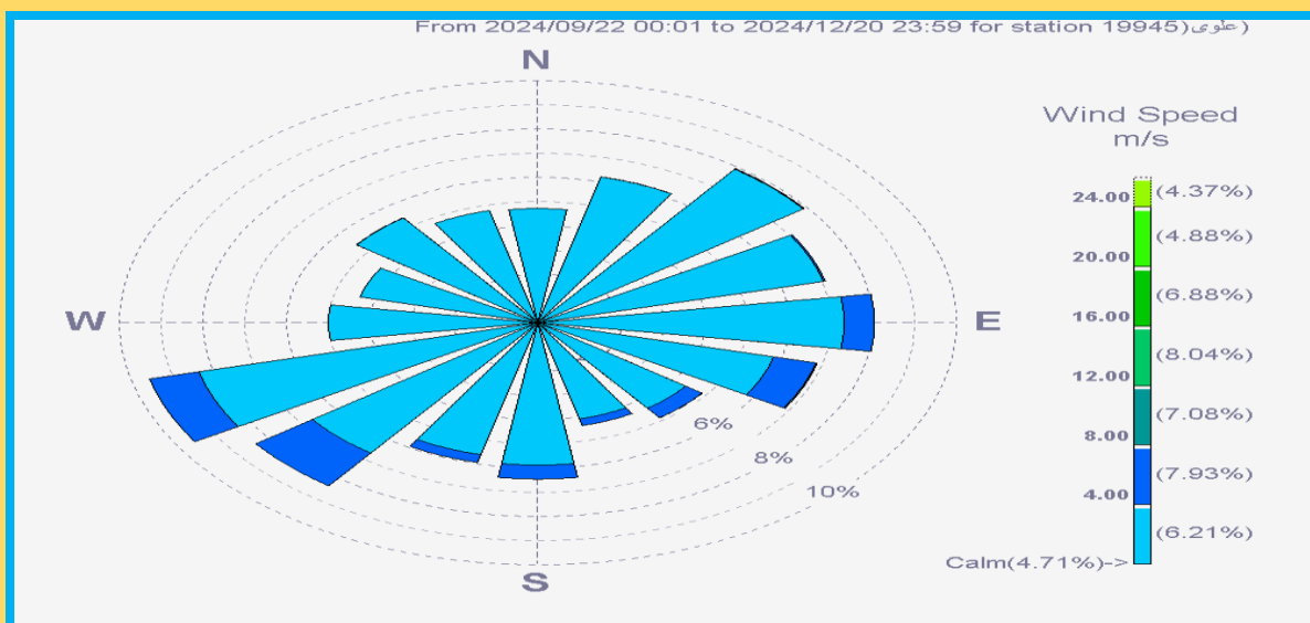
شکل ۴. نمودار گلباد ایستگاه اقلیم شناسی تمام خودکار علوی در فصل پاییز ۱۴۰۳
