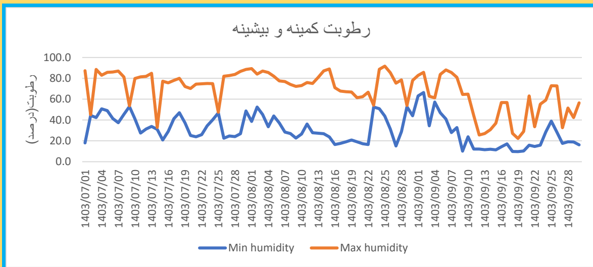
شکل ۳. نمودار سری زمانی رطوبت بیشینه و کمینه در فصل پاییز ۱۴۰۳
