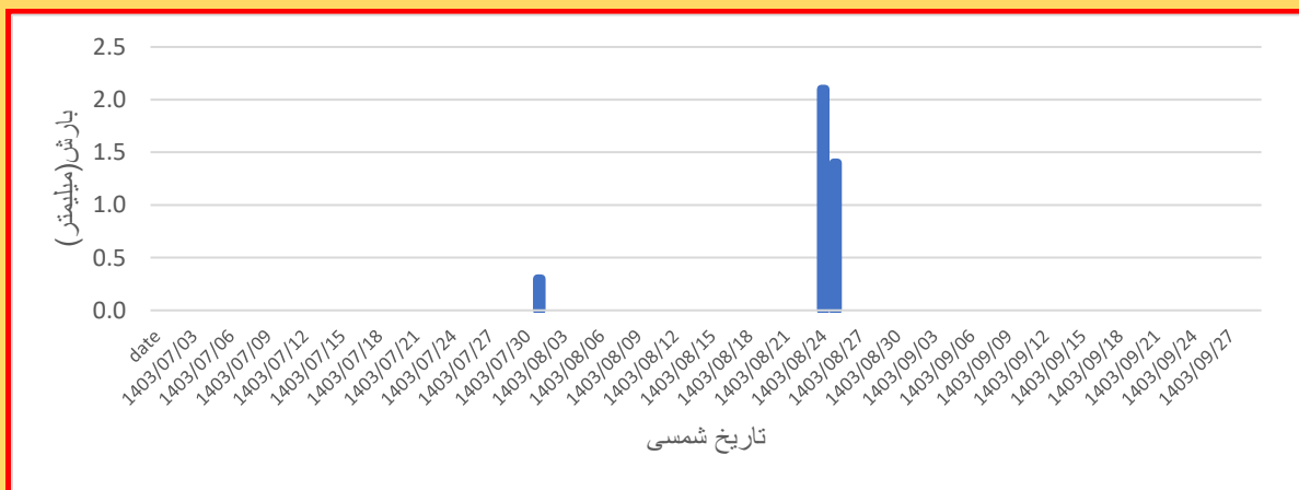
شکل ۲. نمودار میله ای مجموع بارندگی روزانه در فصل پاییز ۱۴۰۳
