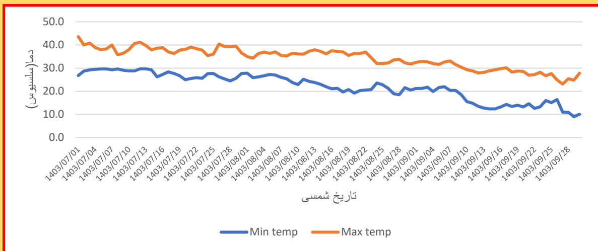
شکل ۱. سری زمانی دمای کمینه و بیشینه در فصل پاییز ۱۴۰۳
