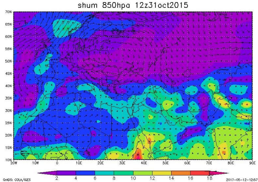
شکل ۲۰- نقشه وزش رطوبتی روز ۳۱ اکتبر تراز ۸۵۰ هکتوپاسکال.
