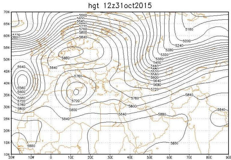
شکل ۱۹- نقشه سطح ۵۰۰ هکتوپاسکال در ساعت ۱۲ UTC روز ۳۱ اکتبر ۲۰۱۵ (ارتفاع بر حسب ژئوپتانسیل متر)
